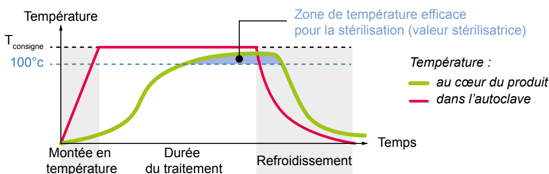
Evolution des températures de l'enceinte et du produit au cours d'un cycle de stérilisation
